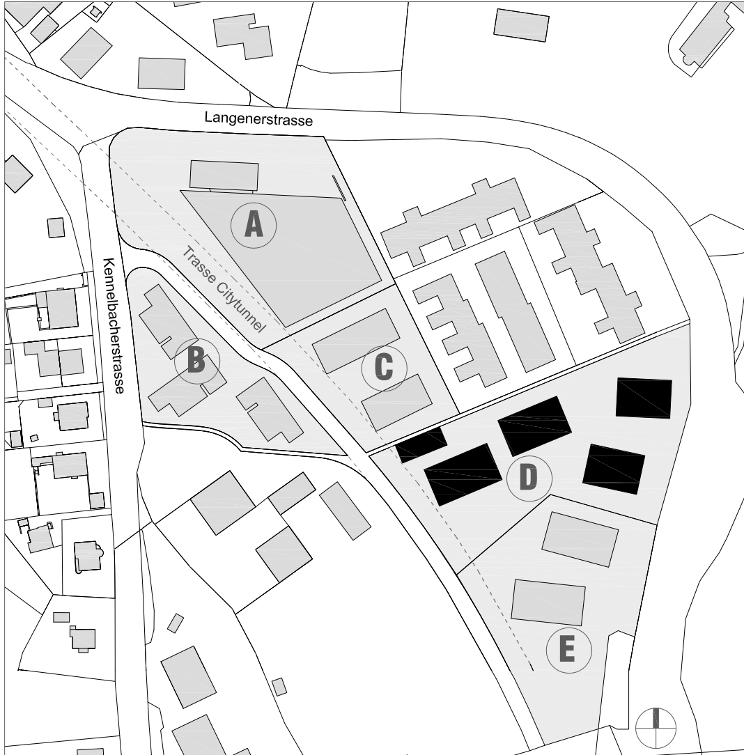
Lageplan
